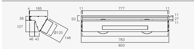
D1010 Diffusore uscita d'aria triplo
