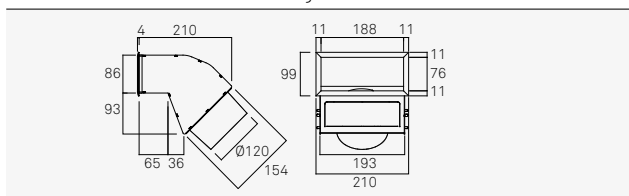
D1002 Diffusore uscita d'aria singolo stretto
