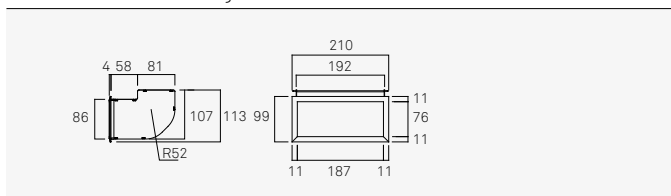
D0002 Presa d'aria singola stretto
