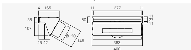
D1005 Diffusore uscita d'aria doppio
