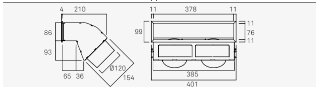
D1007 Diffusore uscita d'aria doppio stretto
