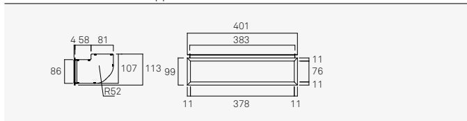
D0007 Presa d'aria doppia stretto
