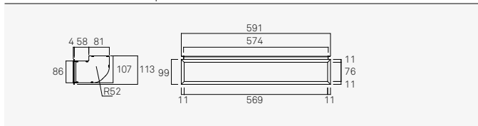
D0015 Presa d'aria quadrupla
