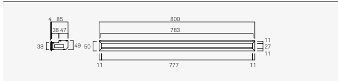
D0010 Presa d'aria tripla
