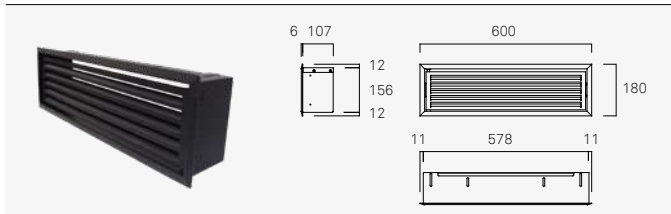
C4000 Presa d'aria accessibile
