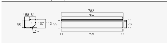
D0015 Presa d'aria quadrupla
