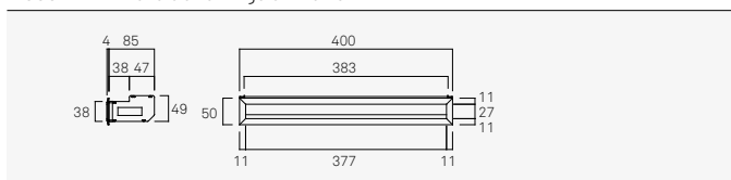
D0005 Presa d'aria doppia
